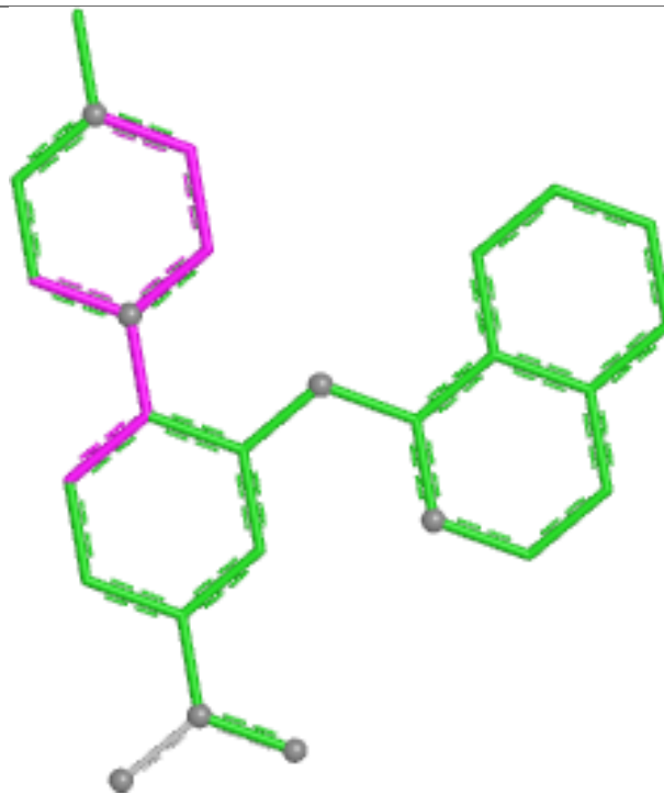
Bond angles
